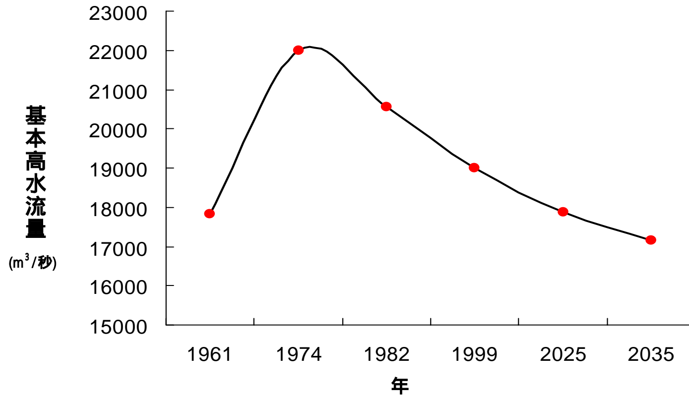
図7 各年度のタンクモデルで推定された基本高水流量(m 3 /s)の推移
